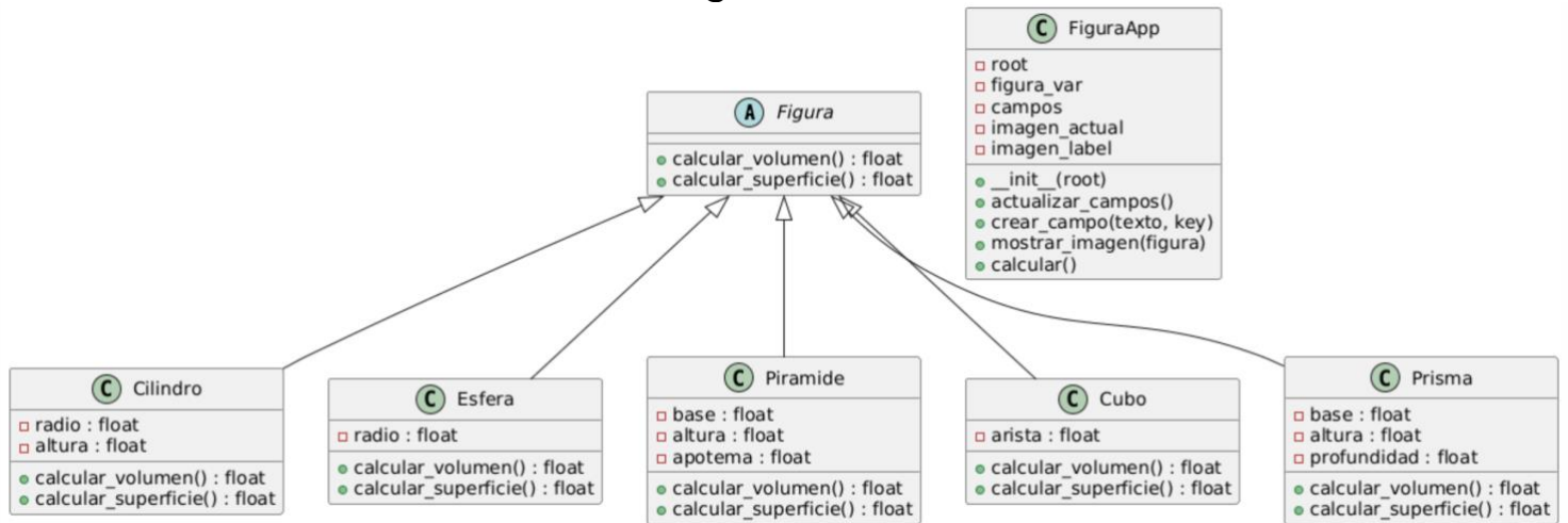
Diagrama UML:
