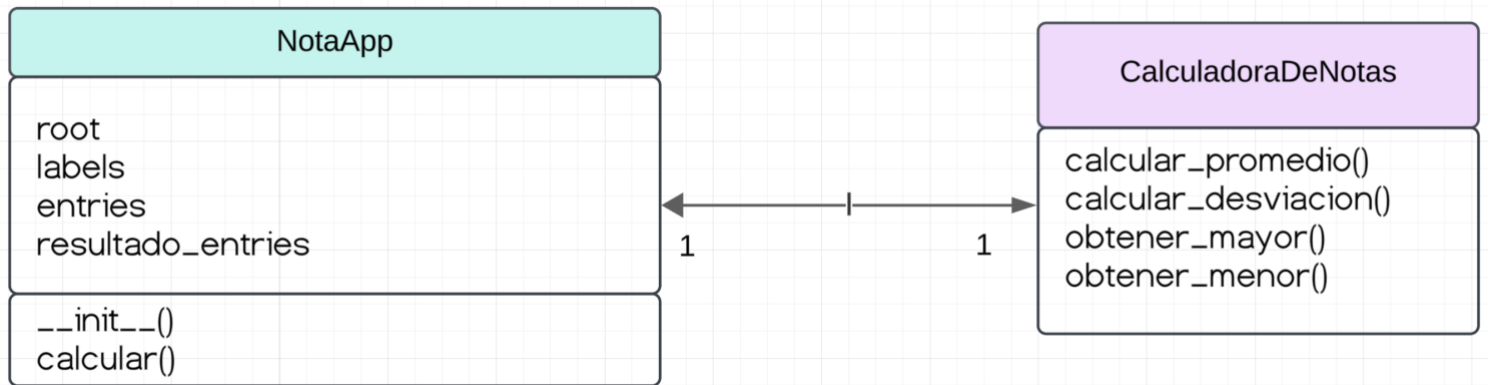
Diagrama UML:
